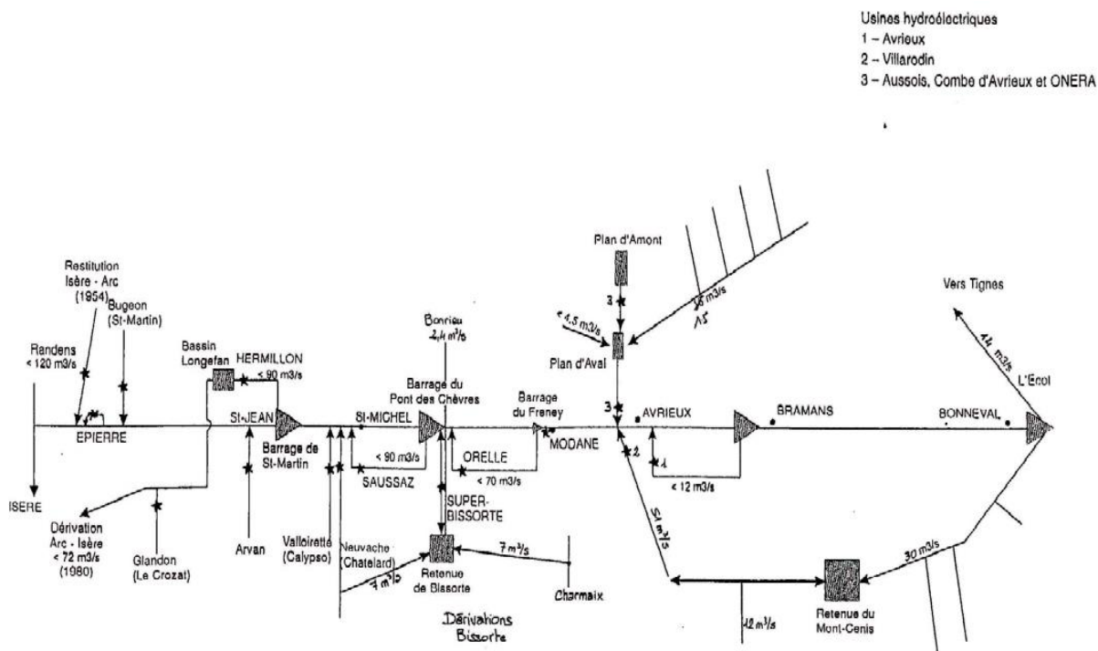
Figure 14 : Schématisation des aménagements hydroélectriques sur le bassin de l'Arc
