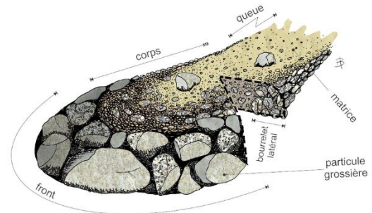
Figure 17 : Schéma de la structure d'une lave torrentielle (www.dsm-consulting.ch)
