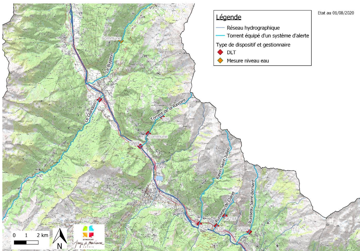
Figure 68 : Dispositifs de prévision des crues et détecteurs de laves torrentielles (DLT)
