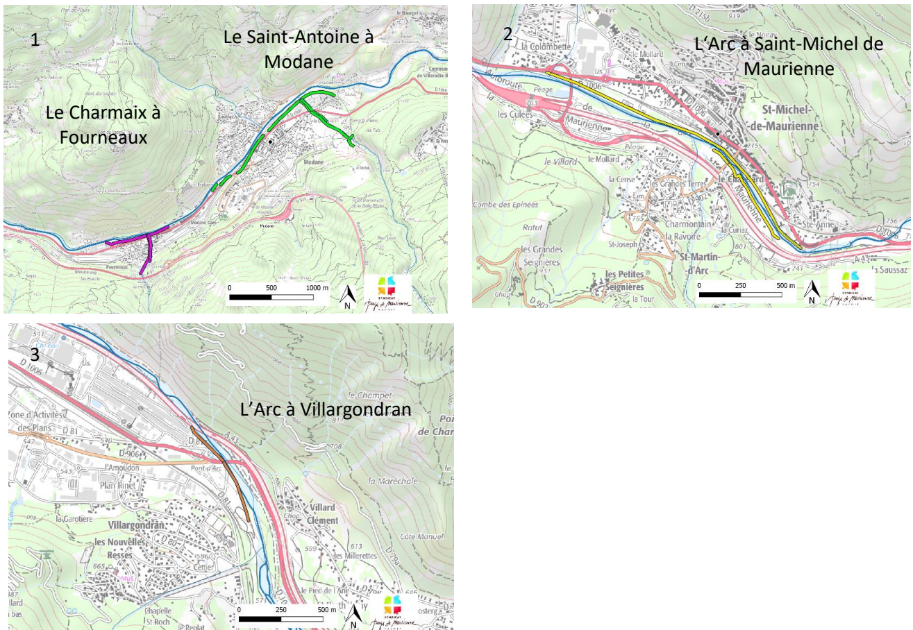
Figure 77 : Localisation des systèmes d'endiguement et zoom sur ceux en classe B
