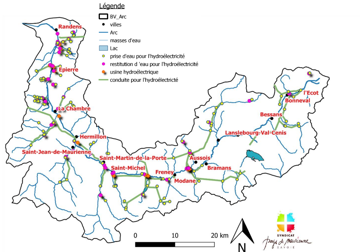
Figure 13 : Aménagements hydroélectriques sur le bassin de l'Arc
